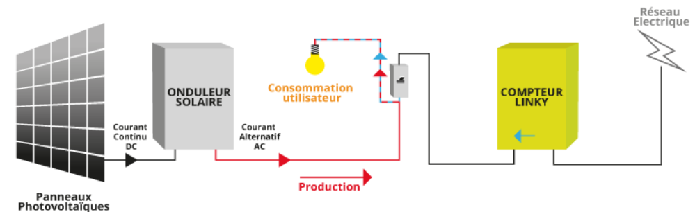
SCHÉMA D'INSTALLATION
